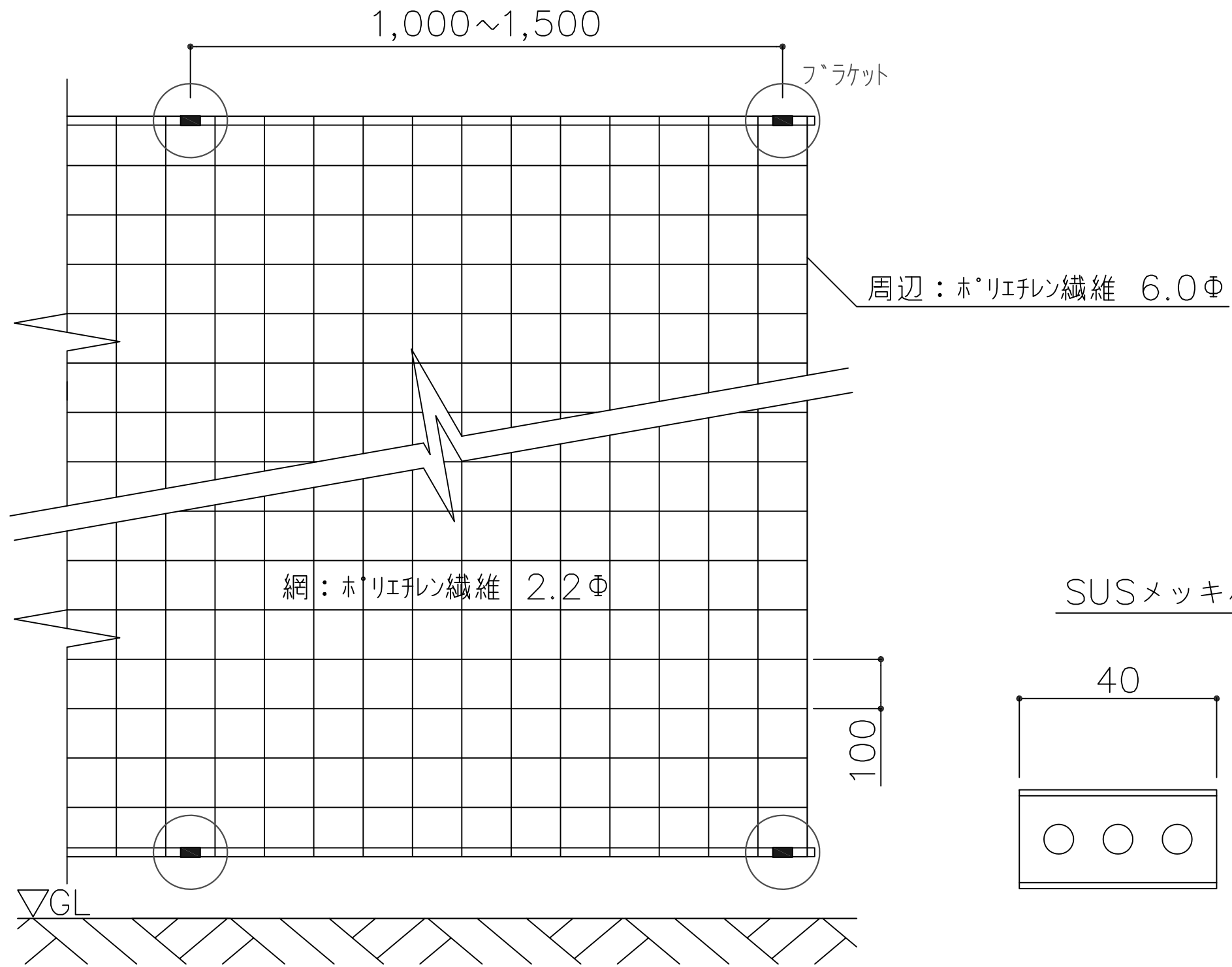
壁面緑化「ひかげ」化繊ネット割付正面図
